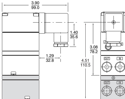
Figure 5 - DIN 43650 Connections
