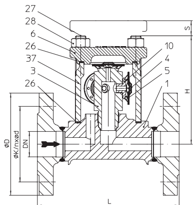
Fig. 616....1....4K2 (DN25) avec 4 capsules, à brides
