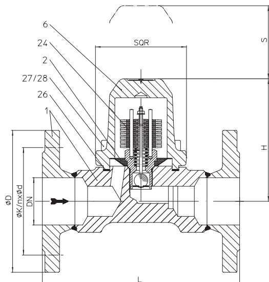
Fig. 600....1 à brides
