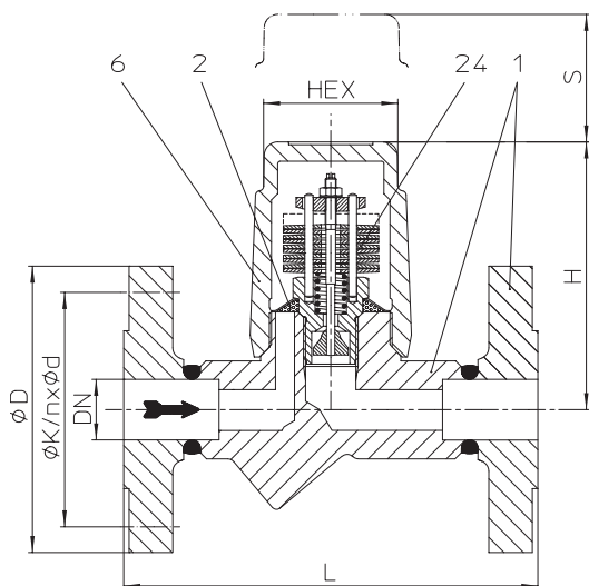
Fig. 600....1 à brides
