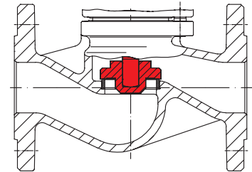
Clapet non attelé (libre) pression différentielle maximale: cf. tableau clapets d'équilibrage. Pression de réponse 0,05 bar Attention: Position de montage droite seulement sur tuyauteries à l'horizontale.
