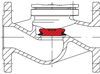
Clapet avec siège à portée conique stellite
