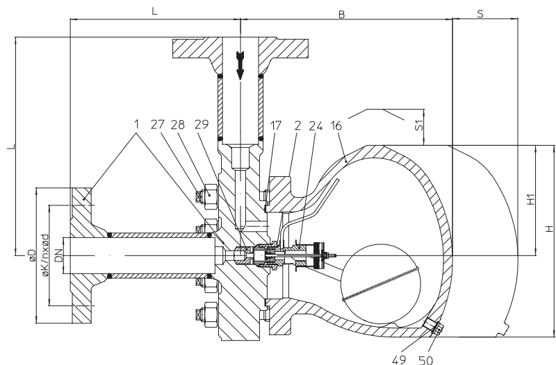
Fig. 632....1 Exécution équerre à brides - montage vertical
